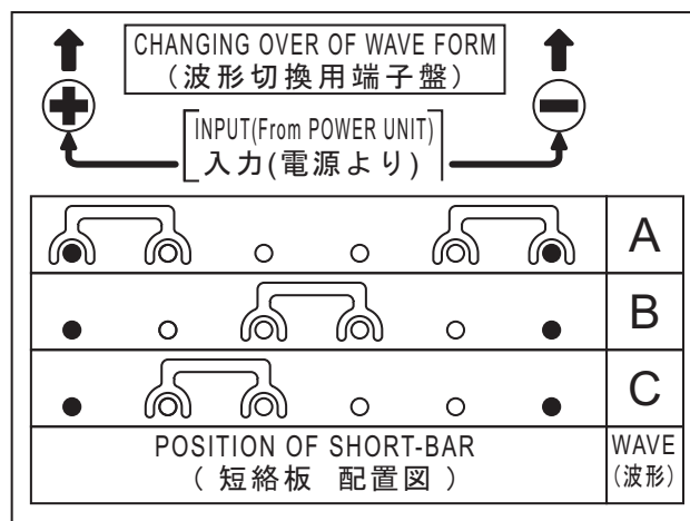
トランスによる波形切換
