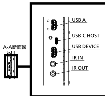
端子部拡大図 a
